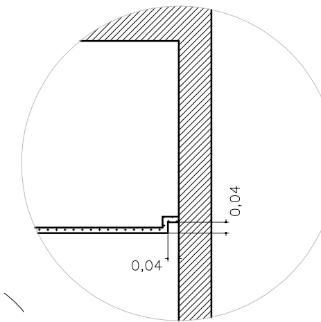
DETALLE B – FOSEADO DE 4 X 4 CMS EN FALSO TECHO. ESCALA 1/20
